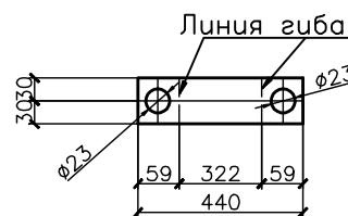
Развертка поз.5
